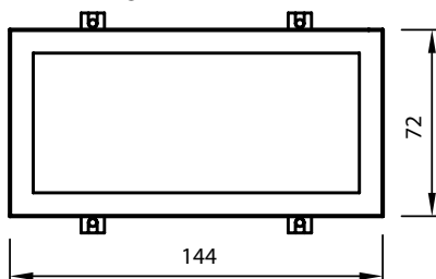
Maattekening A
